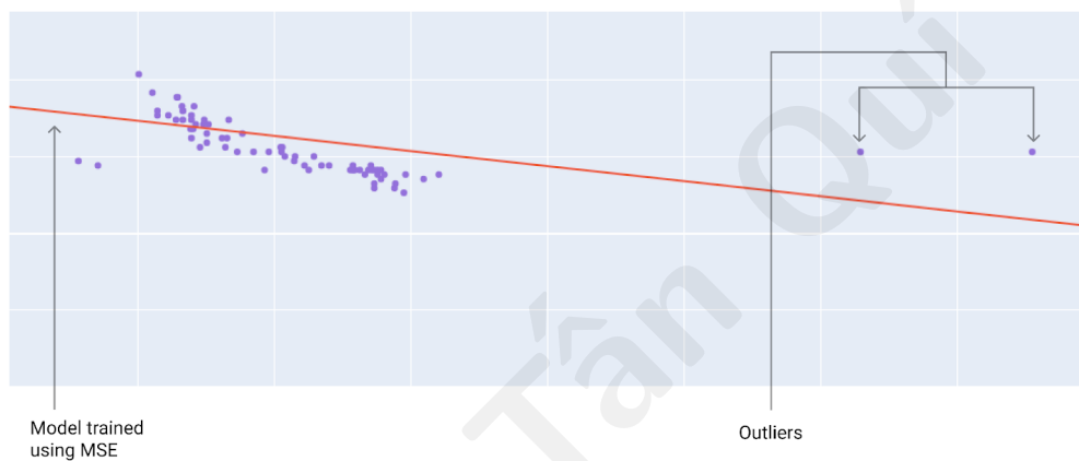
Hình 9. Huấn luyện với MSE — đường (đỏ) gần outlier hơn.
