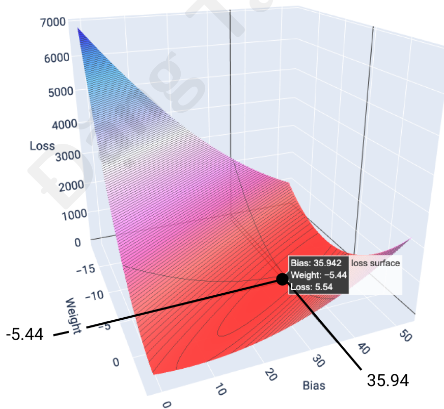
Hình 20. Cực tiểu: w \approx -5,44 , b \approx 35,94 , MSE \approx 5,54 .
